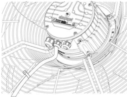
Fig. 2: Liggande monterad fläkt, kablarna dragen så att en droppkant uppstår.
