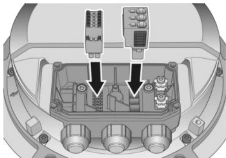
Fig. 2: Montera kontaktdonet i kopplingsdosa
