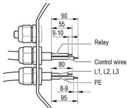
Fig. 1: Rekommenderade skalningslängder i mm (i kopplingsdosa)
